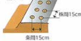
図4 トンネルべた掛け
